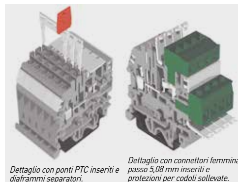
Dettaglio con ponti PTC inseriti e diaframmi separatori. Dettaglio con connettori femmina passo 5,08 mm inseriti e protezioni per codoli sollevate.
