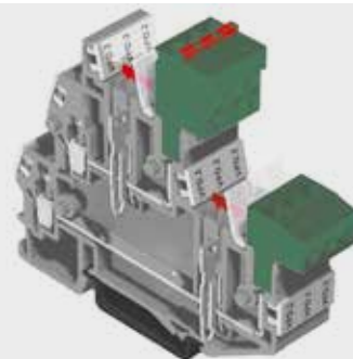
Dettaglio con connettori femmina passo 5,08 mm inseriti sui due livelli e protezioni per codoli sollevate e ponti PTC inseriti sui due livelli.
