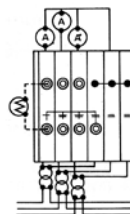
PROVA T.A. TRIFASE CONCATENATO
